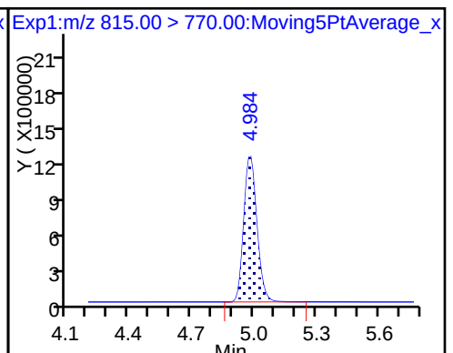
D 44 13C2-PFHxDA
