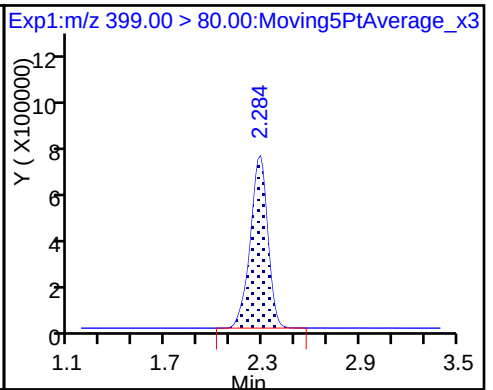
D 12 M2-6:2FTS
