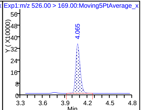
D 43 13C2-PFTeDA
