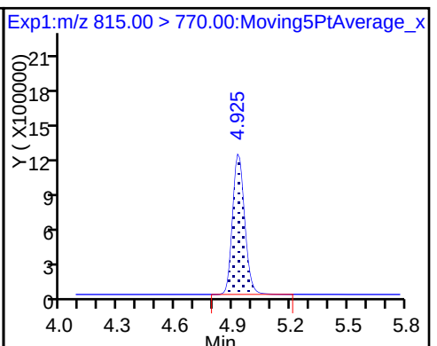
D 44 13C2-PFHxDA
