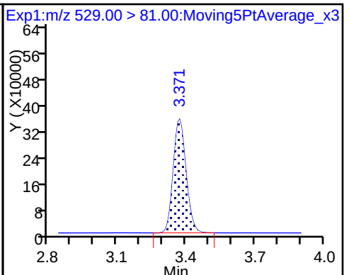
D 26 M2-8:2FTS
