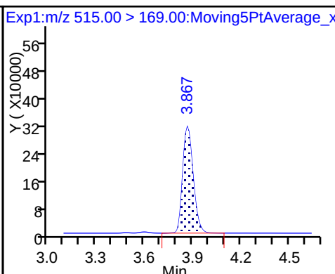
D 34 d-N-MeFOSA-M
