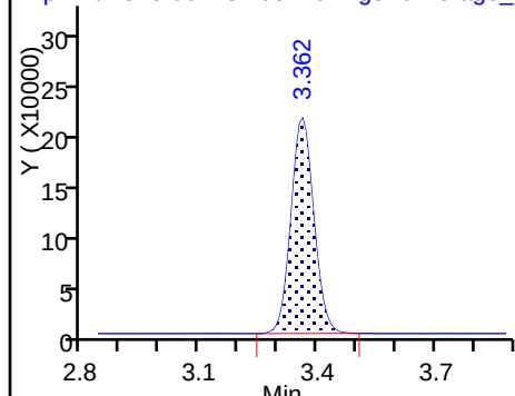
D 26 M2-8:2FTS
