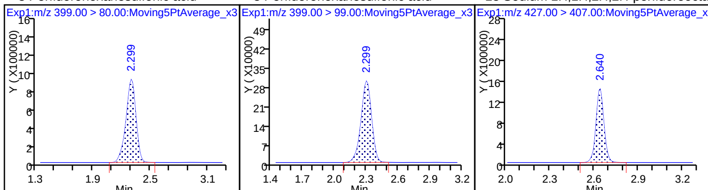
D 12 M2-6:2FTS
