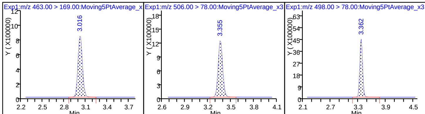
D 26 M2-8:2FTS
