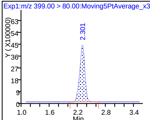
D 12 M2-6:2FTS
