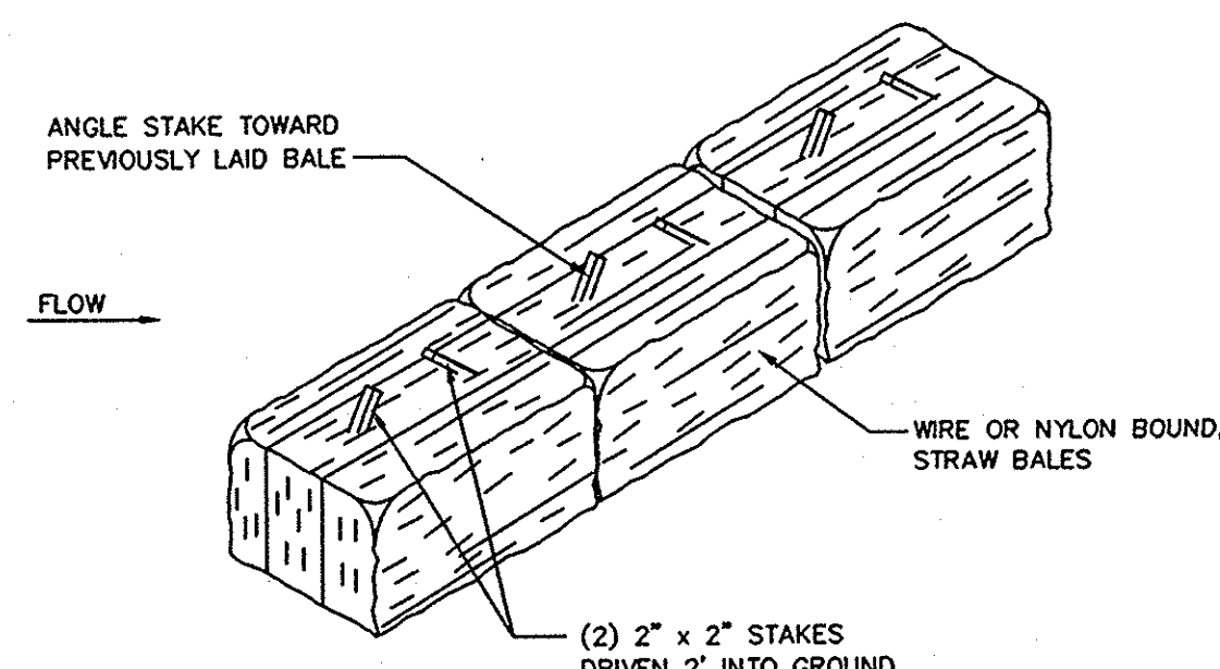
STRAW BALE DETAILS N.T.S.
