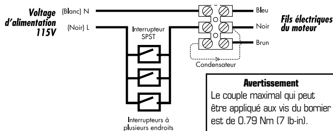
Câblage Romex - Vue de dessus
