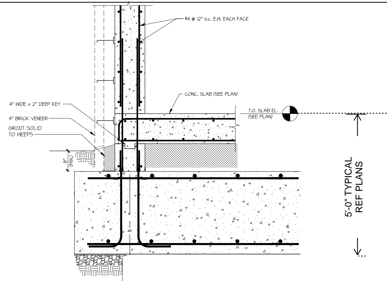
3 SECTION SCALE: 3/4"=1'-0"
