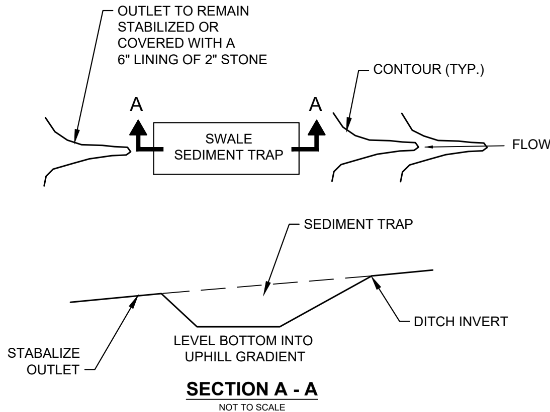
4 SWALE SEDIMENT TRAP SCALE: NTS
