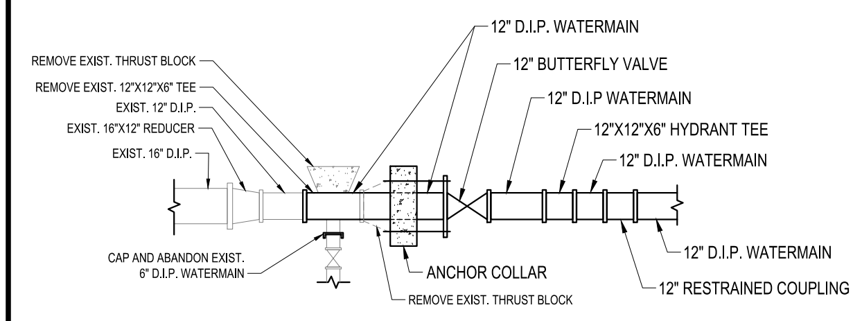
INTERCONNECTION DETAIL #2 SCALE: N.T.S.
