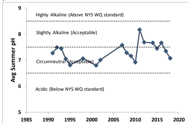
pH
