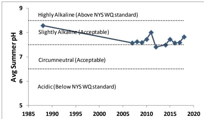
pH
